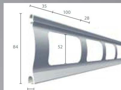
Extrudált alumínium perforált profil
