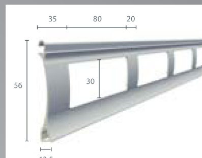
Extrudált alumínium perforált profil
